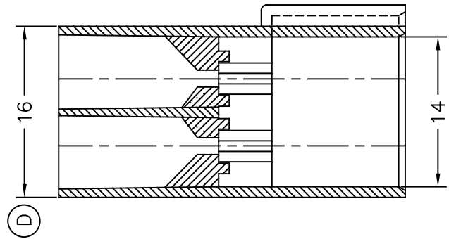
Secc. A-A
